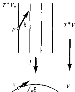
Figure 166 The 1-form p dq on the cotangent bundle
